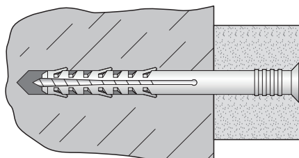
PRZYKŁAD MONTAŻU Installation example
