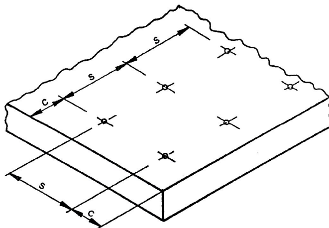
Rysunek B1. Parametry rozmieszczenia łączników rozporowych KAXDN, KAXN i KAXK w podłożu s – rozstaw osiowy łączników, c – odległość łącznika od krawędzi podłoża
