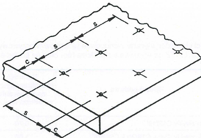
Rysunek B5. Parametry rozmieszczenia łączników tworzywowych LEK, LFK, LEH i LFH w podłożu s – rozstaw osiowy łączników, c – odległość łącznika od krawędzi podłoża
