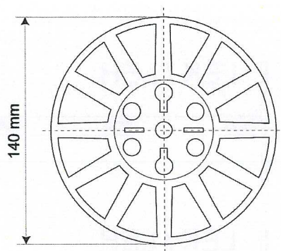
Rysunek A3. Dodatkowy talerzyk TK 140
