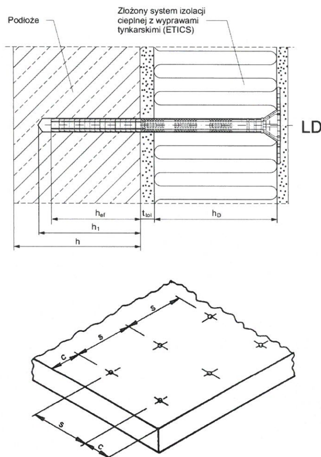
Rysunek B1. Parametry montażu i rozmieszczenia łączników tworzywowych LDK
