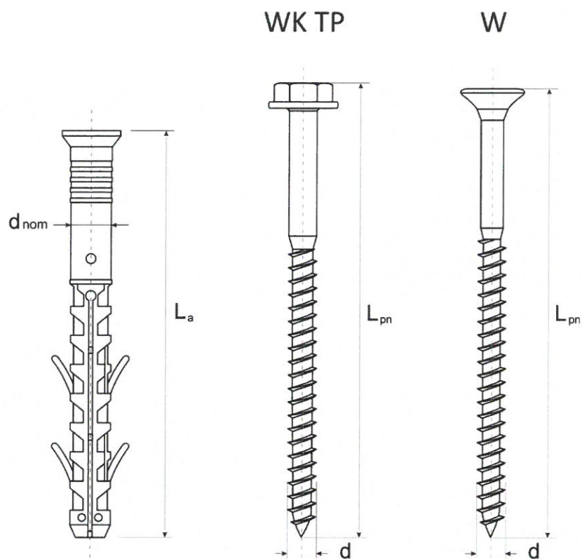
Rysunek A5. Tworzywowo-metalowe łączniki rozporowe KRK 8 TP i KRS 8
