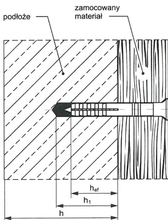
Rysunek B2. Parametry montażu łączników rozporowych KSMK 6 S, KSMK 8 S, KSMN 6 S i KSMN 8 S
