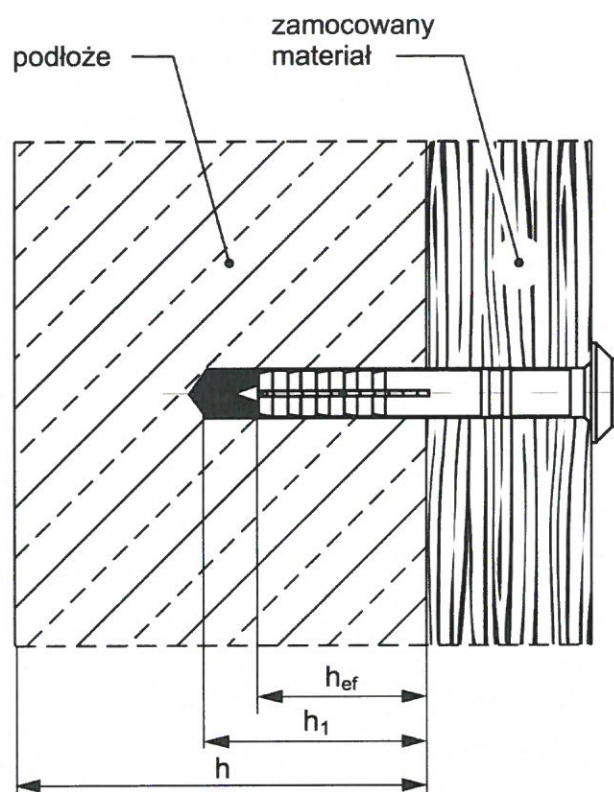
Rysunek B1. Parametry montażu łączników rozporowych KSMK 6 K, KSMK 8 K, KSMN 6 K i KSMN 8 K
