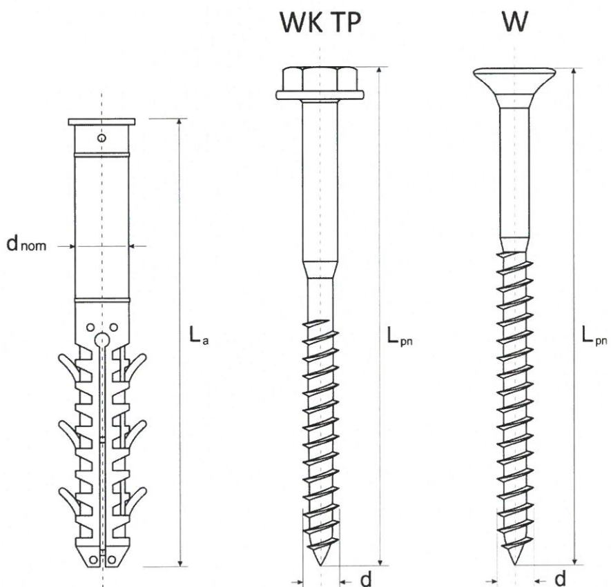
Rysunek A8. Tworzywowo-metalowe łączniki rozporowe KRK 14 TP i KRS 14
