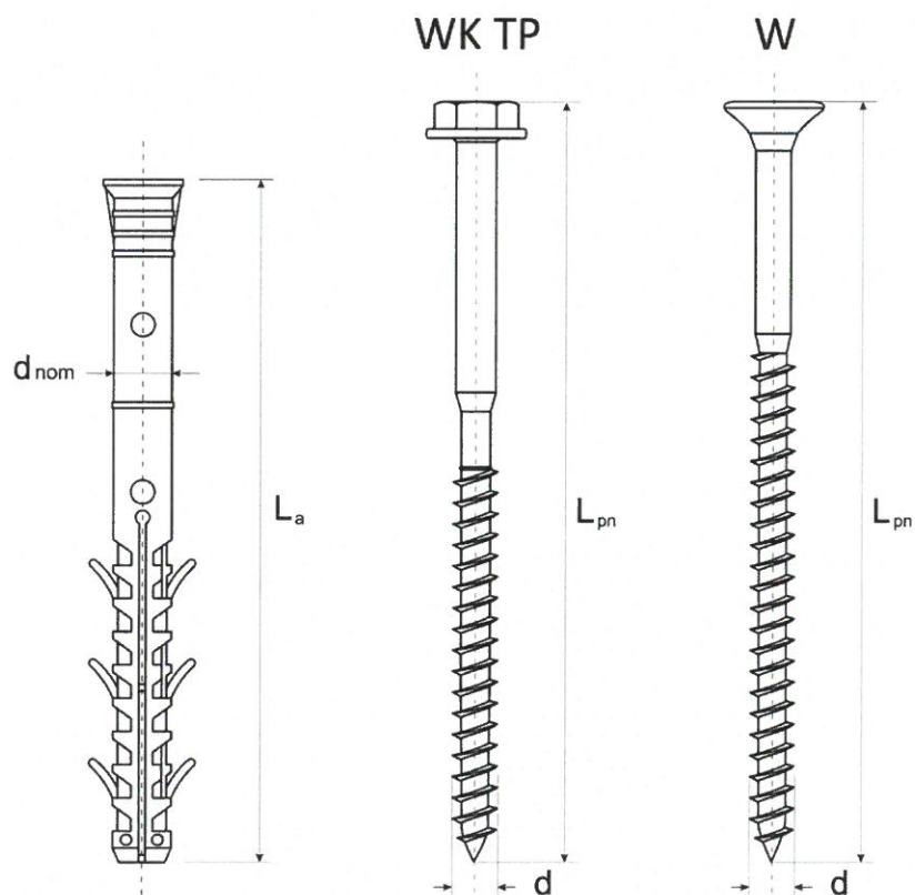
Rysunek A6. Tworzywowo-metalowe łączniki rozporowe KRK 10 TP i KRS 10
