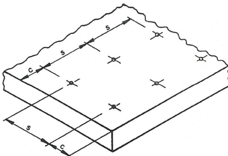
Rysunek B9. Parametry rozmieszczenia łączników rozporowych KSMK, KSMN, KRK TP i KRS w podłożu s – rozstaw osiowy łączników, c – odległość łącznika od krawędzi podłoża
