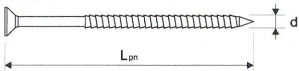
Rysunek A2. Tworzywowo-metalowe łączniki rozporowe KSMK 6 S i KSMN 6 S
