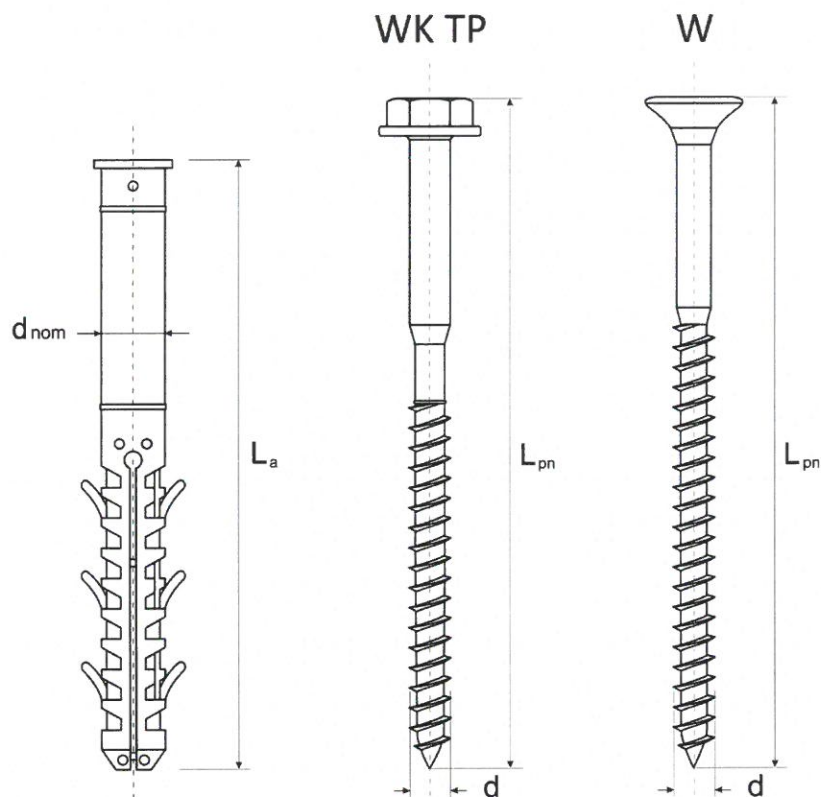
Rysunek A7. Tworzywowo-metalowe łączniki rozporowe KRK 12 TP i KRS 12
