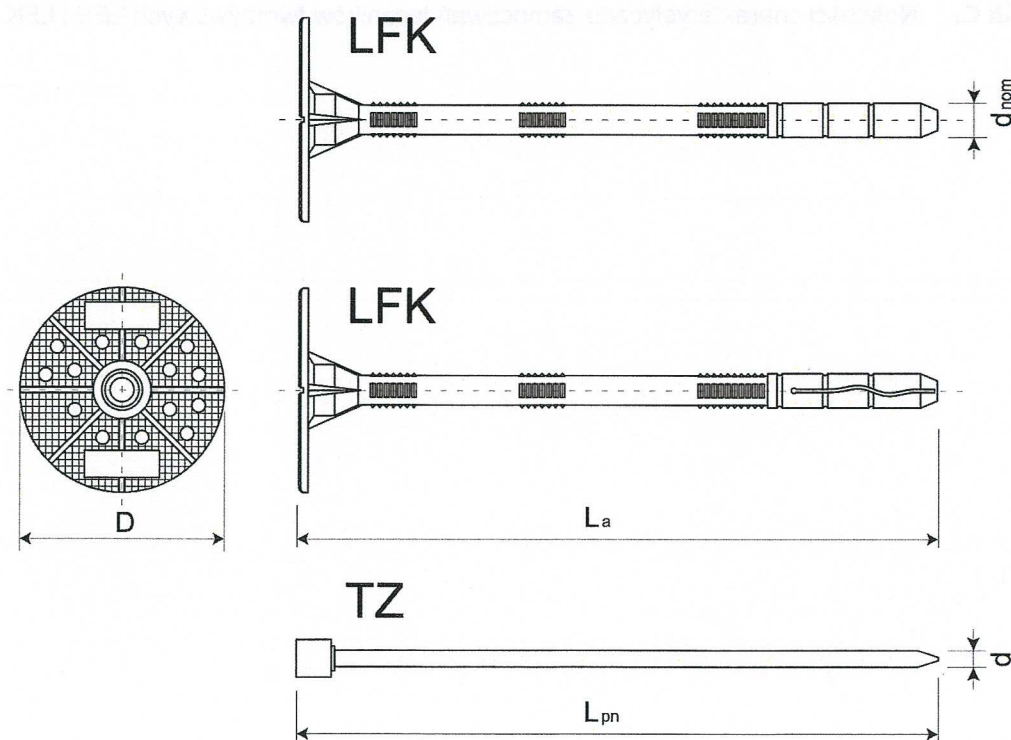
Rysunek A2. Łącznik tworzywowy LFK
