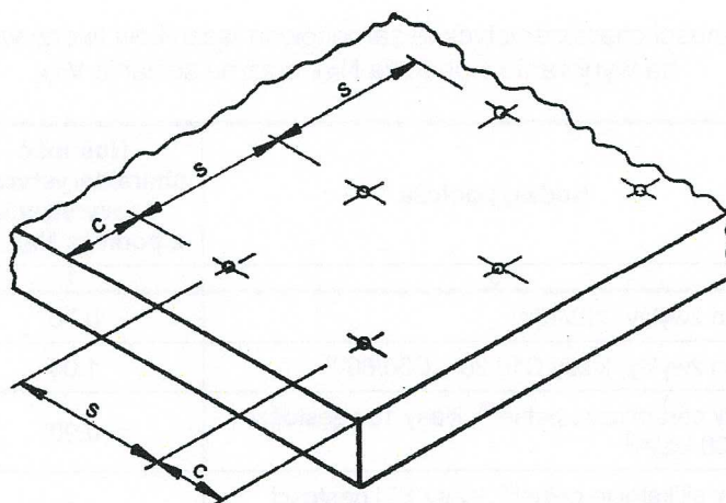
Rysunek B2. Parametry rozmieszczenia łączników tworzywowych LEK i LFK w podłożu s – rozstaw osiowy łączników, c – odległość łącznika od krawędzi podłoża
