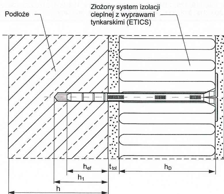
Rysunek B1. Parametry montażu łączników tworzywowych LFK
