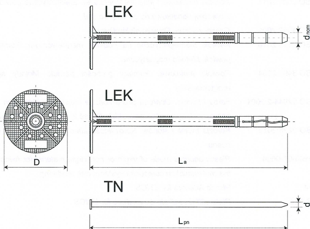
Rysunek A1. Łącznik tworzywowy LEK
