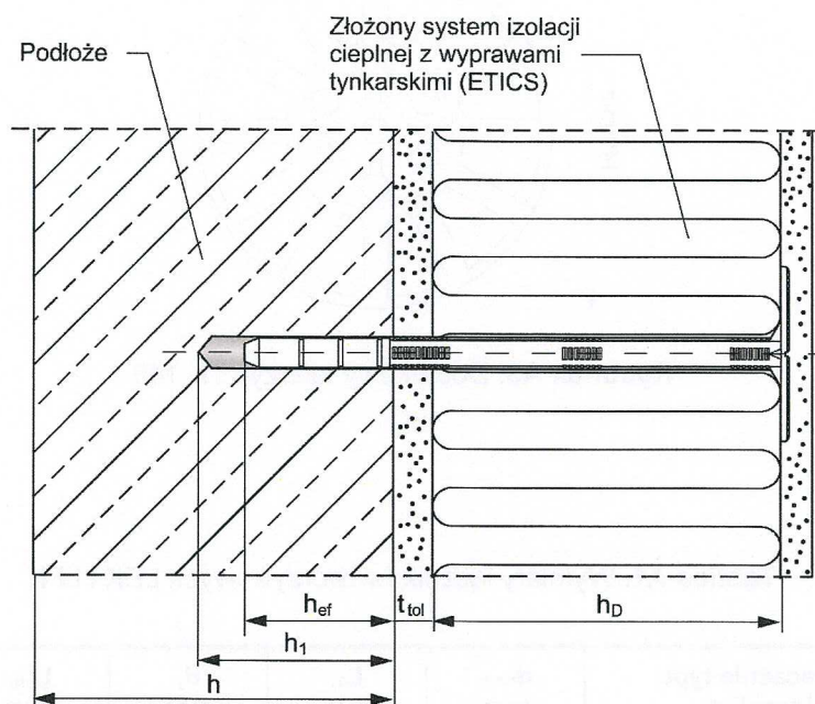
Rysunek B1. Parametry montażu łączników tworzywowych LEK
