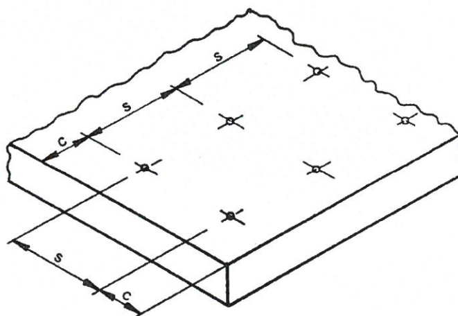
Rysunek B2. Parametry rozmieszczenia łączników tworzywowych LX w podłożu s – rozstaw osiowy łączników, c – odległość łącznika od krawędzi podłoża
