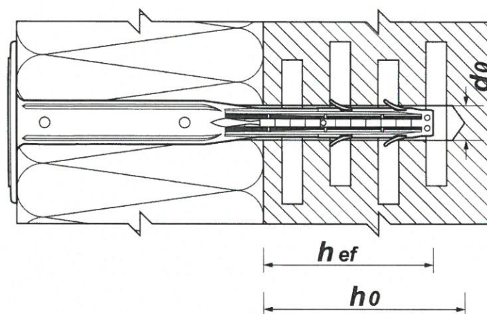
Rysunek B1. Parametry montażu łączników tworzywowych LX
